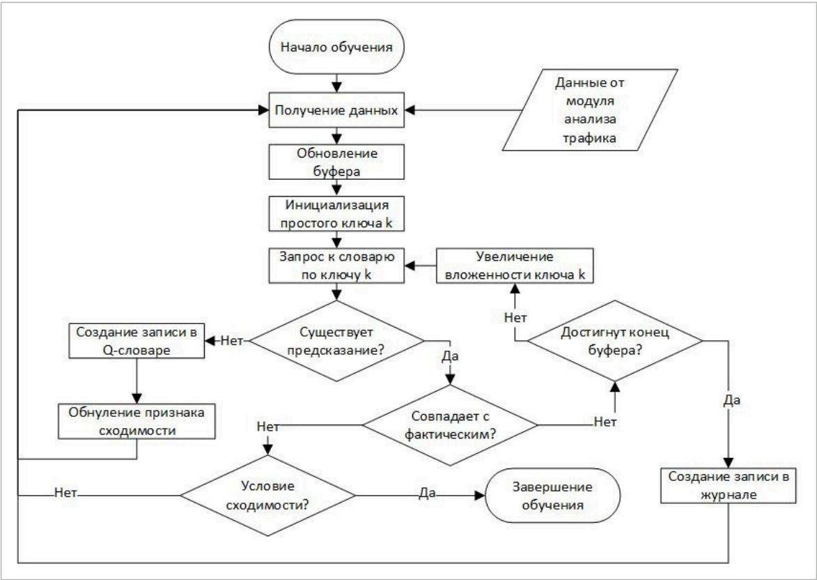
Рис. 569. Схема обучения модели на основе иерархического словаря
