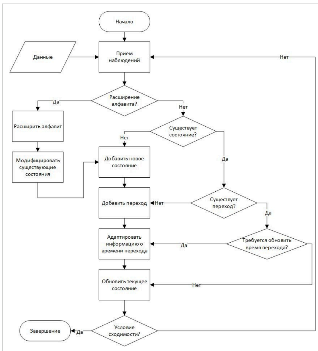
Рис. 570. Схема обучения модели на основе временного автомата
